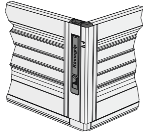
Montante e profilo connessione Montante chiuso
